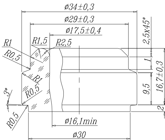
Венчик горловины тип III ГОСТ 10117.2-2001
